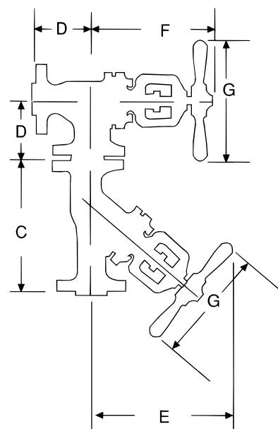
1643/1641 Angle Globe
